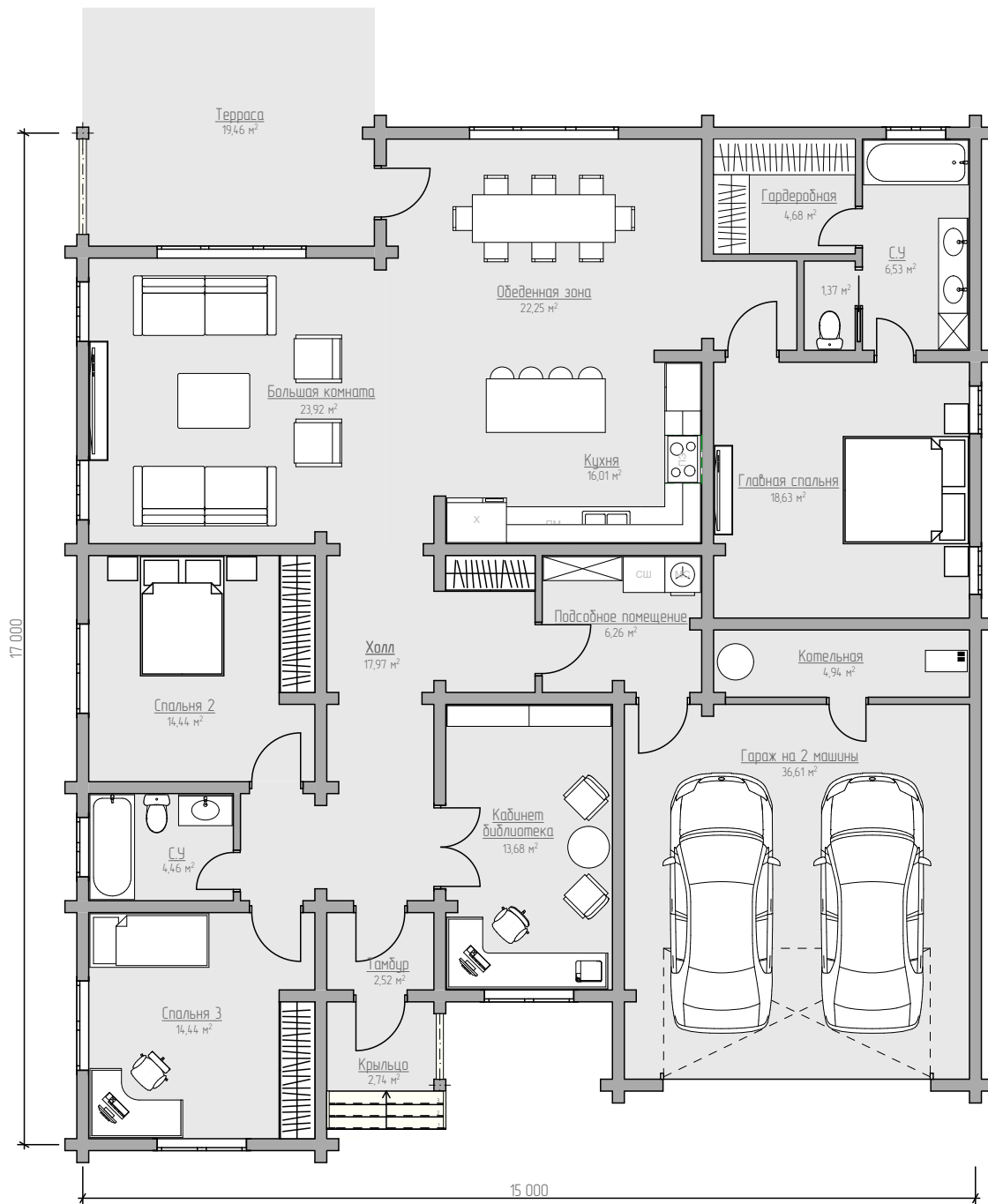
План одноэтажного дома
